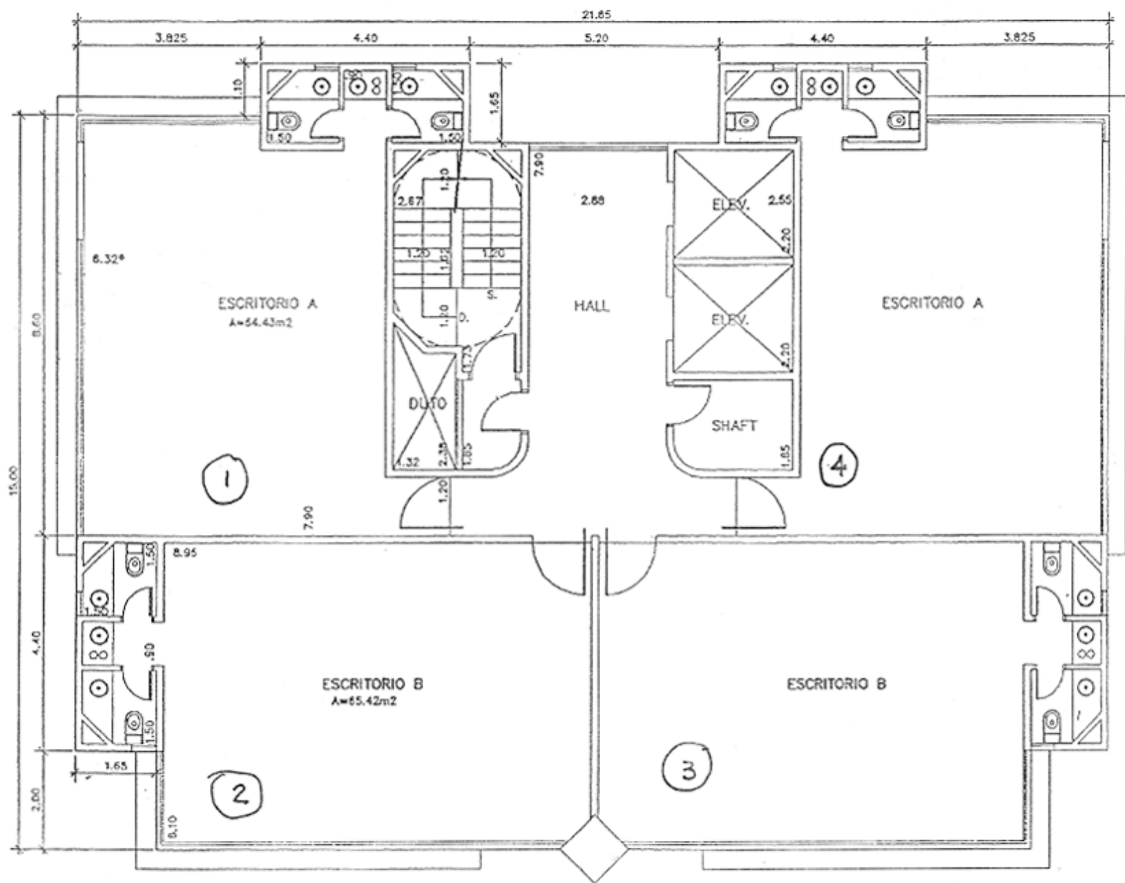
PLANTA PAV. TIPO (1° ao 13°)
